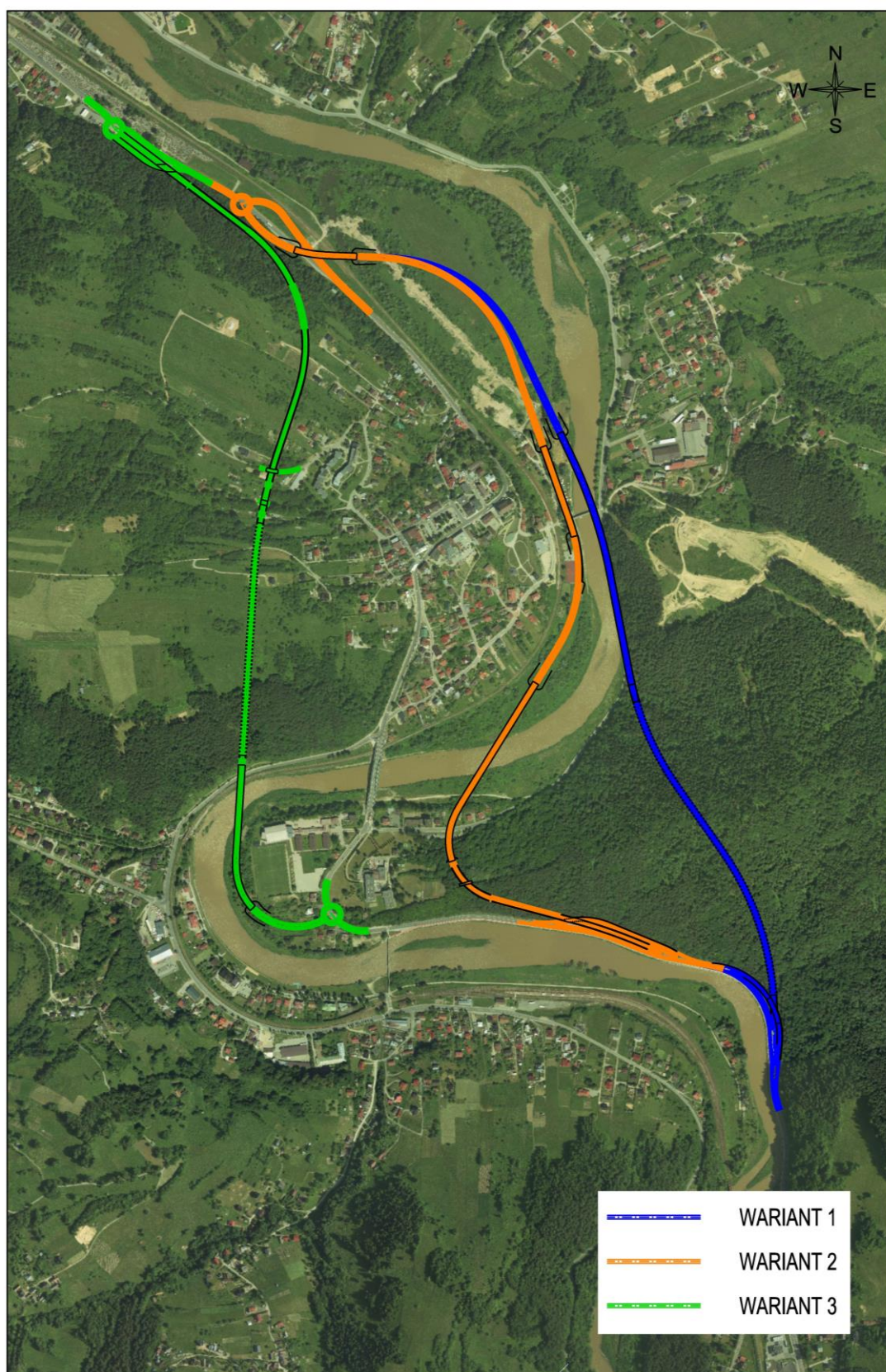
Rysunek 4. Plan orientacyjny przebiegu trzech wariantów obwodnicy Piwnicznej-Zdroju w ciągu DK nr 87 źródło: GDDKiA
