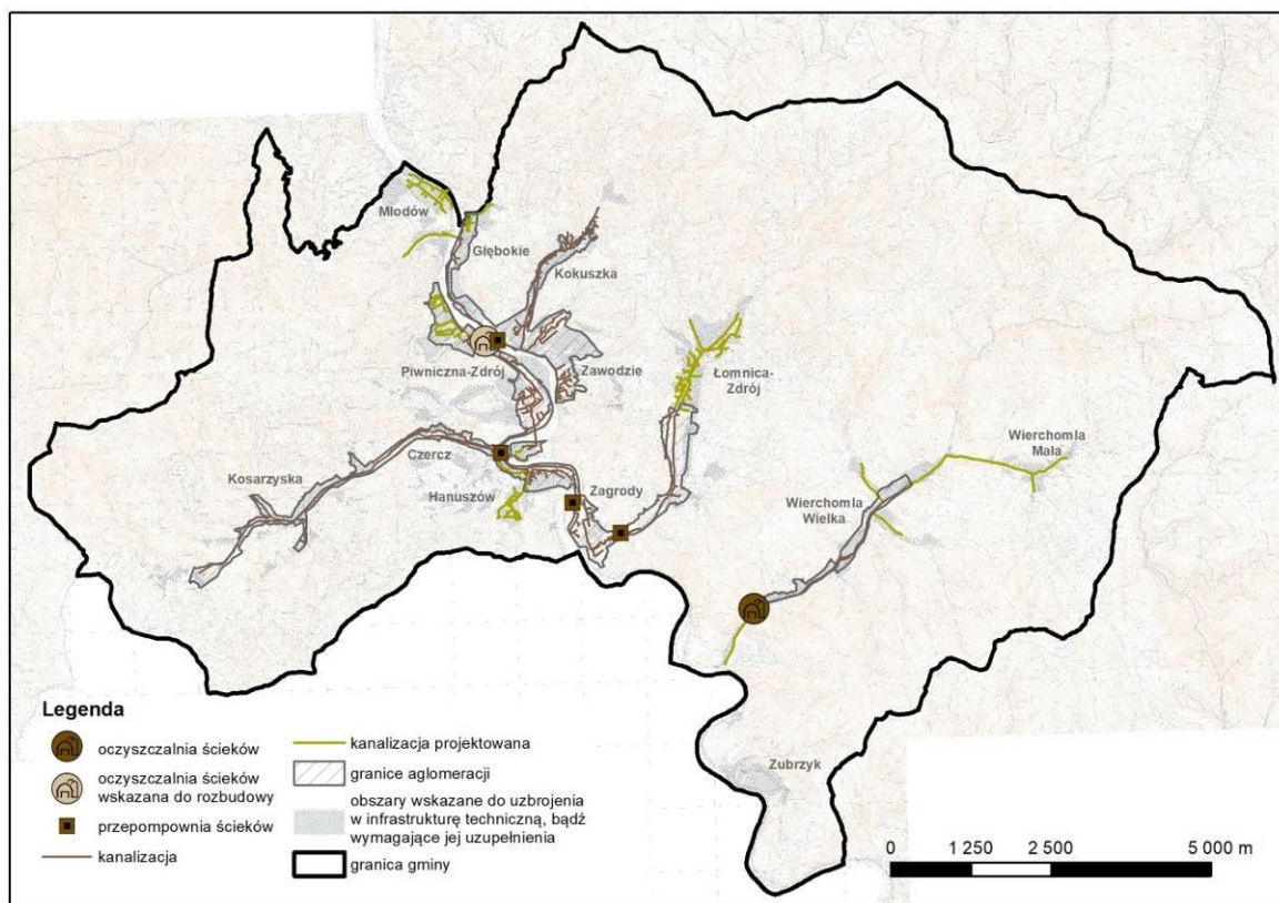
Rysunek 26. Kierunki rozwoju sieci kanalizacyjnej
