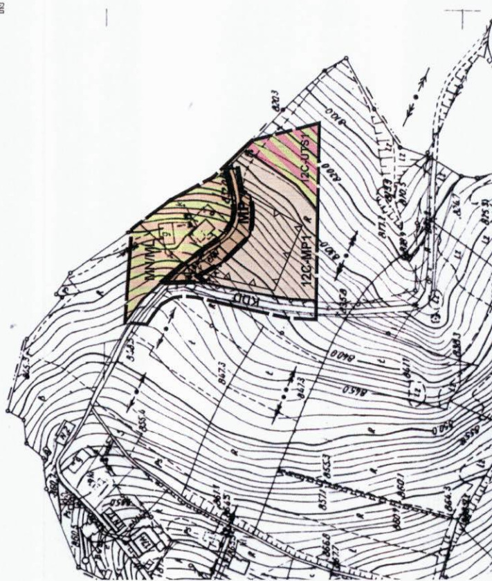
RYSUNEK PLANU
